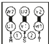
Conexión de motores Estrella/triángulo
