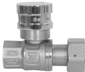
VÁLVULA MONTADA CON TAPÓN ANTIFRAUDE Y LLAVE MAGNETICA PARA EL DESBLOQUEO DEL TAPÓN ANTIFRAUDE
