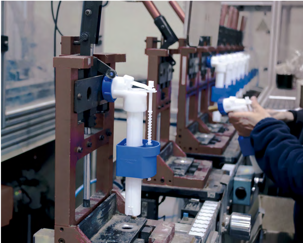
ESTACIÓN DE COMPROBADO GRIFOS SERVO
