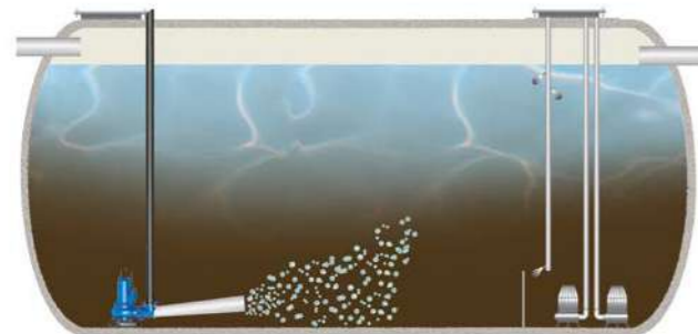
Dibujo Homogeneizador especial con turbina
