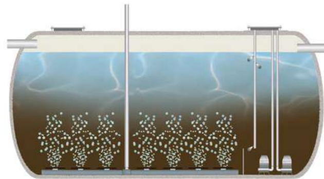
Dibujo Homogeneizador estándar con difusores
