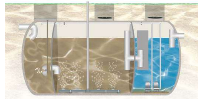
REACTOR ANÓXICO REACTOR AIREADO DECANTADOR SECUNDARIO
