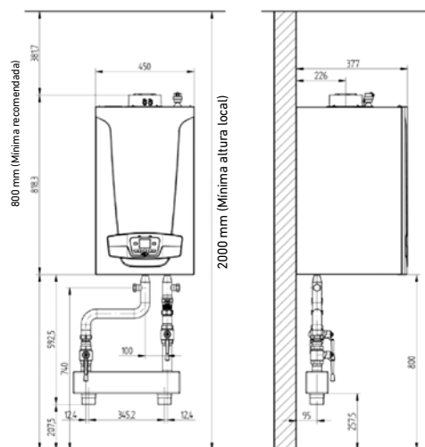
Bios Plus 50 F y 70 F
