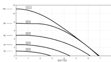
WGB 50 (circulador opcional)
