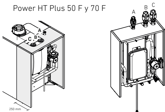
Kit botella de equilibrio
