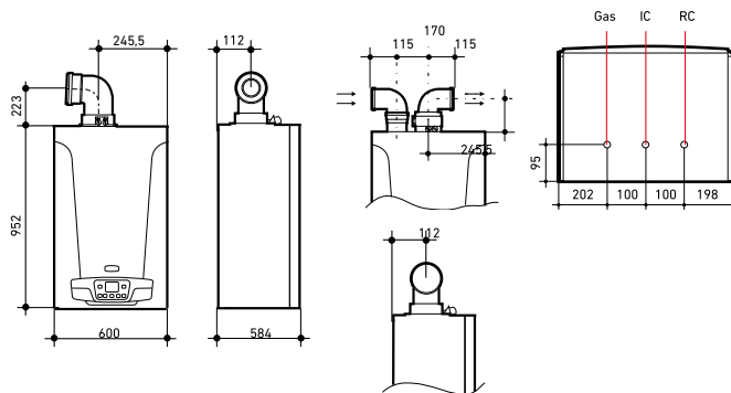
Bios Plus 90 F, 110 F, 130 F y 150 F
