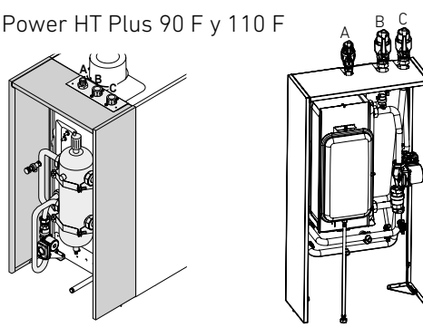
Kit botella de equilibrio
