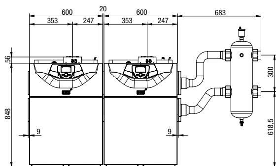
Power HT Plus 50 F y 70 F
