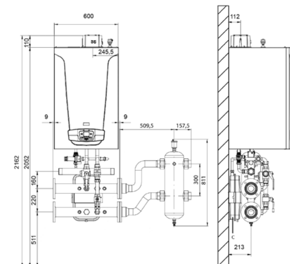
Bios Plus 90 F, 110 F, 130 F y 150 F
