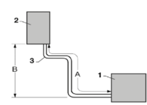
1. Unidad Exterior 2. Unidad Interior 3. Número máximo de codos: 15 Usar un radio de curvatura de 100 mm
