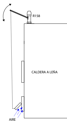
Instalación vertical
